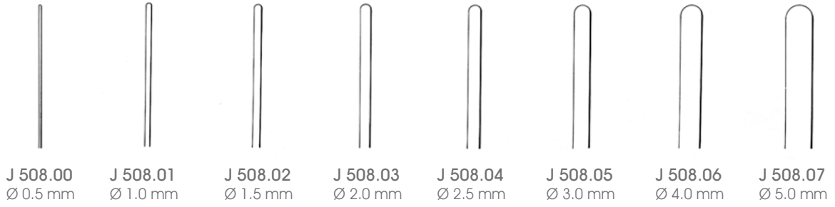
COOLEY J 508.00 - J 508.07 Bükülebilir/Malleable 13 cm
